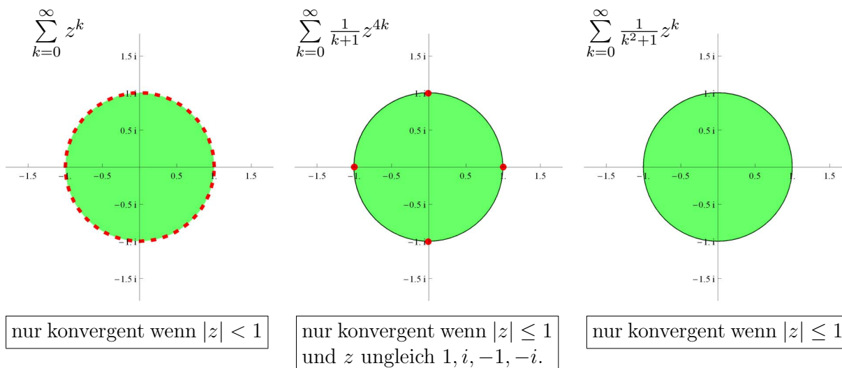
Abbildung 8.1: Konvergenzgebiete
