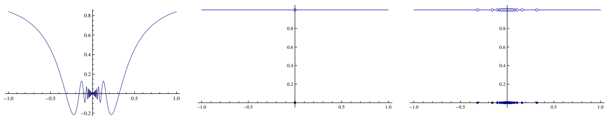
Abbildung 10.1: Skizzen zu g , f und f(g) .
