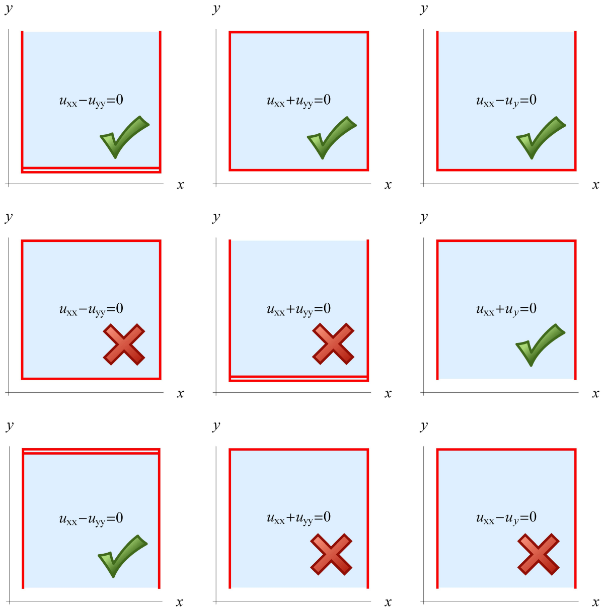
Abbildung 5.8: Ein roter Strich bedeutet, dass man einen Randwert vorschreibt. Bei zwei Strichen braucht es einen zweiten unabhängigen Randwert. Es gibt wohl-definierte (✓) und nicht-wohl-definierte Probleme (✗) im Sinne von Hadamard. Zu der Aussage in fast jedem dieser Beispiele gehört ein nicht-trivialer Beweis.
