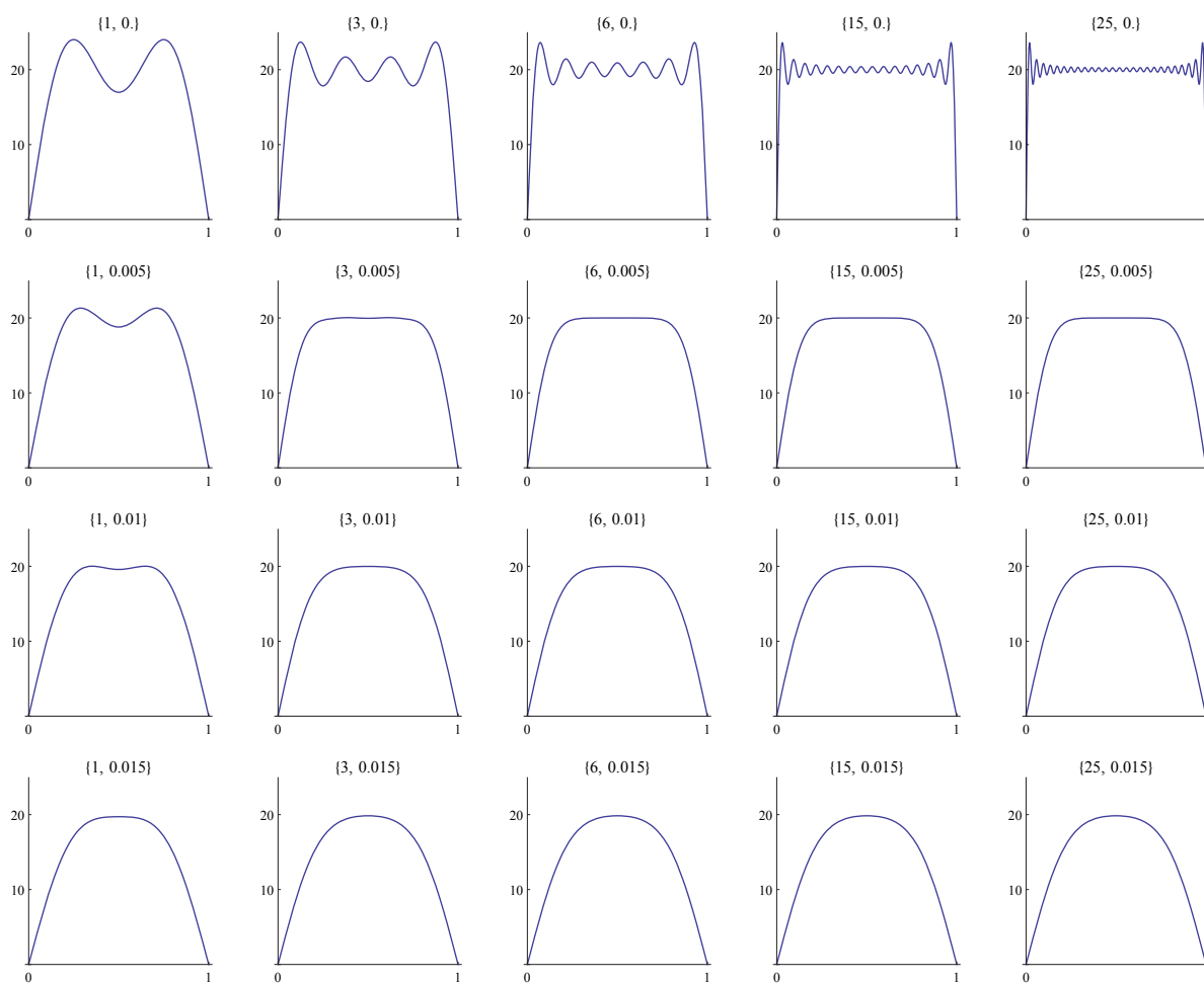
Abbildung 5.6: Skizzen einiger Funktionen die (5.18) approximieren, wo \infty ersetzt ist durch n , für n \in \{1, 3, 6, 15, 25\} und für fest gewählte t \in \{0, 0.005, 0.01, 0.015\} . Nach rechts ist n zunehmend; nach unten wird t größer.
