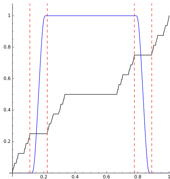
Abbildung 2.1: Die monotone Cantorfunktion und eine geschickt gewählte Testfunktion.
