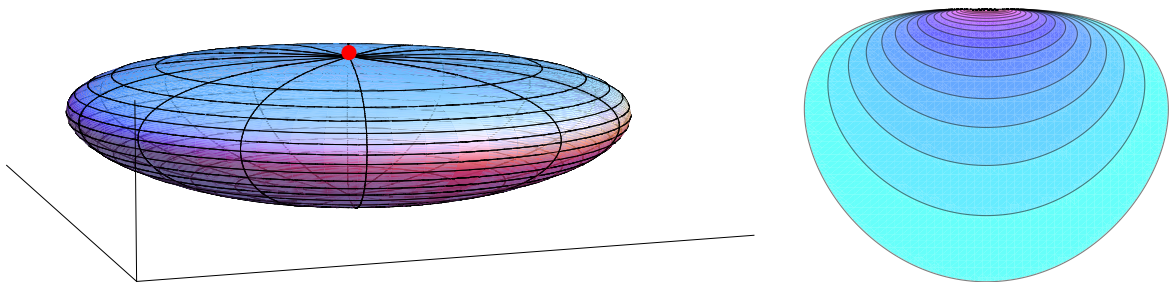
Abbildung 9.3: Links eine Wärmeleitungskugel W(x, t, r) in \mathbb{R}^2 \times \mathbb{R} mit dem Punkt (x, t) in rot. Rechts mehrere solchen Kugeln in \mathbb{R} \times \mathbb{R} .
