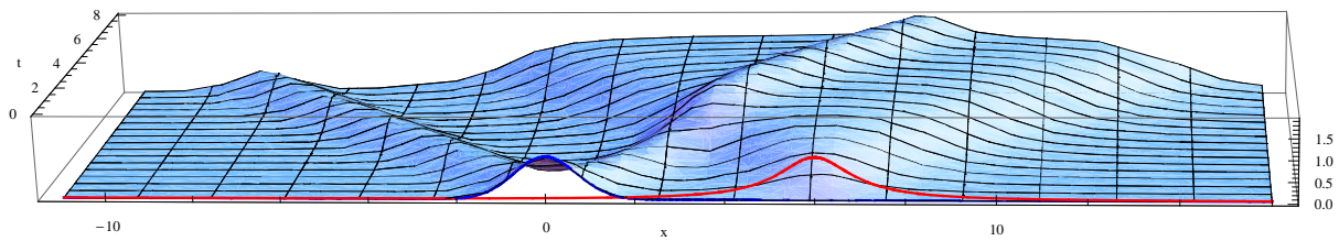
Abbildung 6.1: Skizze der Lösung nach d'Alembert von (6.2) mit c = 1 und u_0(x) = e^{-x^2} (in blau) und v_0(x) = \frac{1}{1+(x-6)^2} (in rot).
