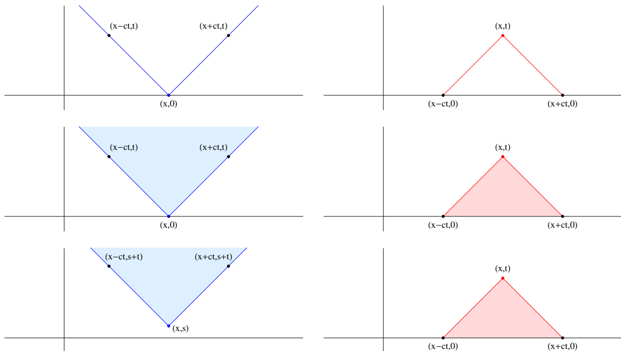
Abbildung 6.3: Oben: Das Einflussgebiet und das Abhängigkeitsgebiet zu u_0 . Mitte: Der Einflusskegel und der Abhängigkeitskegel zu v_0 . Unten: Der Einflusskegel und der Abhängigkeitskegel zu f .
