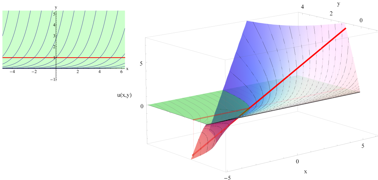
Abbildung 4.2: Skizzen zu Beispiel 4.8. Links oben die charakteristischen Kurven und rechts die Lösung oberhalb der charakteristischen Kurven. In rot ist die Bedingung u(x, 1) = x + 1 dargestellt.
