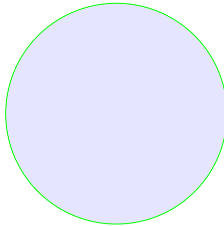
Abbildung 5.4: Rundherum u vorschreiben gibt eine eindeutige Lösung bei -\Delta u = f . Siehe (5.16).
