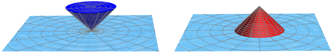
Abbildung 8.3: Einfluss- und Abhängigkeitsgebiet in 2 Dimensionen; die Zeit nach oben und in blau (x, t) \in \mathbb{R}^2 \times \{0\} . Im Gegensatz zu 3 Dimensionen ist der Kegel nun gefüllt.
