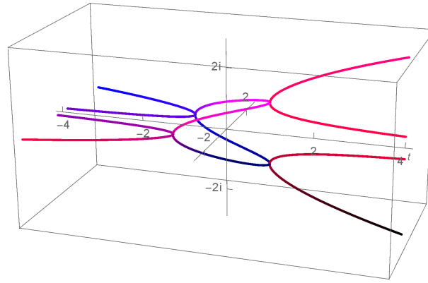
Abbildung 5.9: Die vier Nullstellen t \mapsto \lambda(t) : \mathbb{R} \rightarrow \mathbb{C} von \lambda^4 + 2t\lambda^2 + 1 = 0 als Funktion von t .
