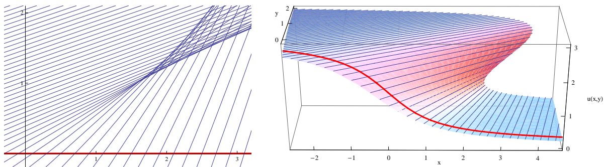
Abbildung 4.3: Skizzen zu Beispiel 4.10. Links die teilweise sich \u00fberschneidenden charakteristischen Kurven und rechts eine Skizze zu den Parametrisierungen (s, t) \mapsto (x(t; s), y(t; s), U(t; s)) . In rot ist die Bedingung u(x, 0) = \frac{1}{2}\pi - \arctan x dargestellt. Die Mannigfaltigkeit (s, t) \mapsto (x(t; s), y(t; s), U(t; s)) l\u00e4sst sich nur bedingt als Graph einer Funktion (x, y) \mapsto u(x, y) darstellen.
