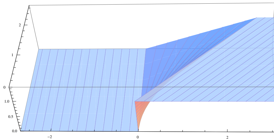
Abbildung 4.8: Eine physikalisch relevante Lösung zu (4.25)-(4.26).
