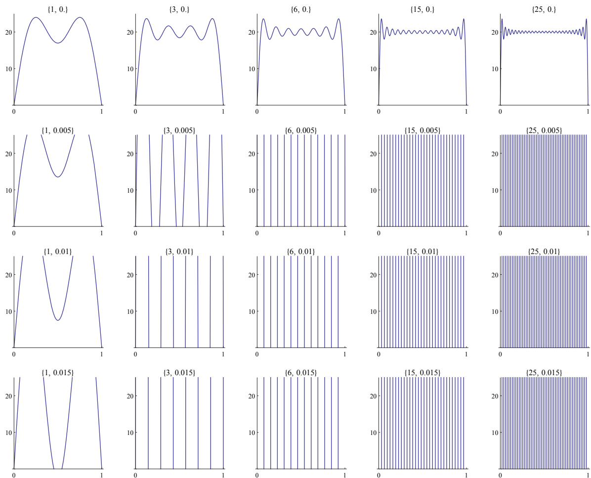
Abbildung 5.7: Skizzen der Funktionen x \mapsto 20 \sum_{k=0}^n \frac{4}{(2k+1)\pi} e^{(2k+1)^2 \pi^2 t} \sin((2k+1)\pi x) für n \in \{1, 3, 6, 15, 25\} und t \in \{0, 0.005, 0.01, 0.015\} . Man vergleiche mit den Bildern in Fig. 5.6.
