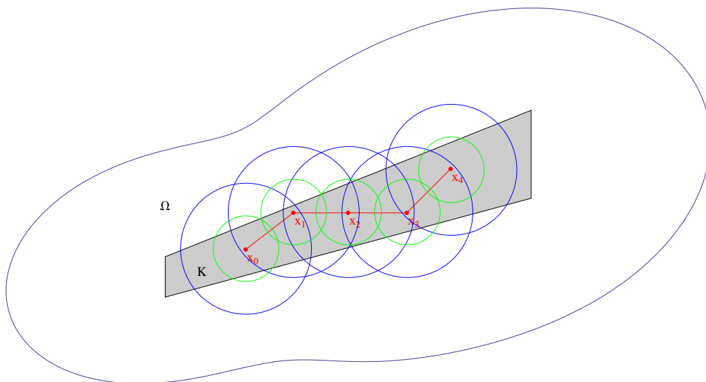
Abbildung 8.3: Skizze zum Beweis der Harnackschen Ungleichung.
