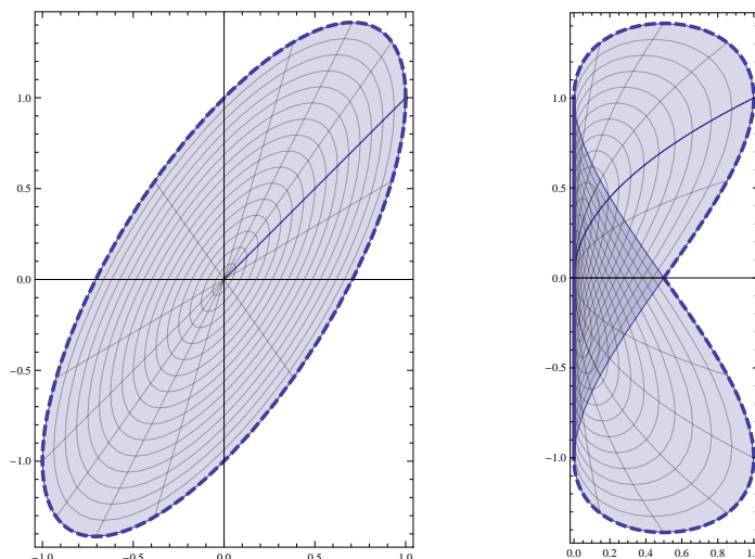
Abbildung 10.3: Rechts das Bild des linken Gebietes unter der Abbildung f aus Bemerkung 10.4.1, die nicht holomorph ist. Das Bild der offenen Ellipse ist nicht offen, da rechts die Gerade zwischen i und -i sowohl in als auch auf dem Rand von h(G) liegt. Die Abbildung ist nicht gebietstreu.
