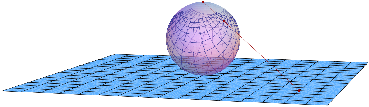
Abbildung 2.8: \mathbb{C} als \mathbb{R}^2 und die Projektion aus (2.9) auf der Einheitskugel um (0, 0, 1) .
