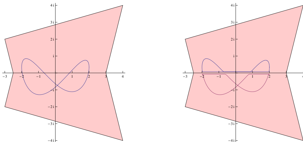
Abbildung 14.3: Die Kurven \gamma und \gamma^+, \gamma^- . Bemerke, dass Teilkurven, die in entgegengesetzten Richtungen durchlaufen werden, sich aufheben und nicht am Integralwert beitragen.
