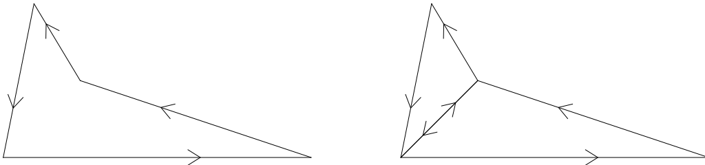
Abbildung 4.1: Rechts mit zusätzlicher Geraden ohne Einfluss auf den Wert des Integrals, weil sie in beiden Richtungen einmal durchlaufen wird.
