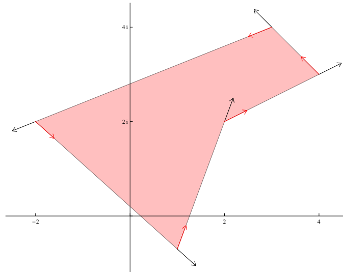
Abbildung 14.4: Die Winkeländerungen erscheinen in der Schwarz-Christoffel Transformation. Im Bild ist \alpha_k der Winkel vom schwarzen zum roten Vektor an der Stelle w_k .
