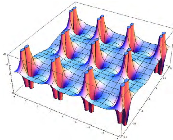
Abbildung 13.9: Skizze zu \text{Re}(\varphi(\cdot; p_1, p_2)) .
