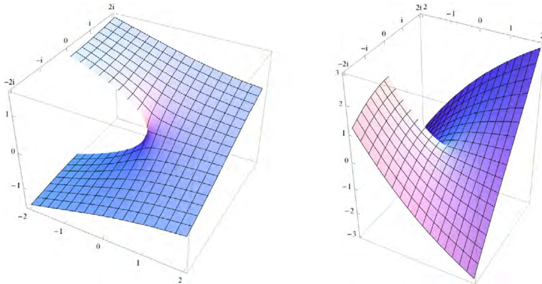
Abbildung 5.4: Links eine Skizze der Funktion z \mapsto \text{Im}(\sqrt{z}) und rechts z \mapsto \text{Im}\left(\frac{2}{3}z\sqrt{z}\right) . Man sieht die Unstetigkeit auf \mathbb{R}^- .
