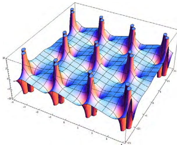
Abbildung 13.10: Skizze zu \text{Im}(\varphi(\cdot; p_1, p_2)) .
