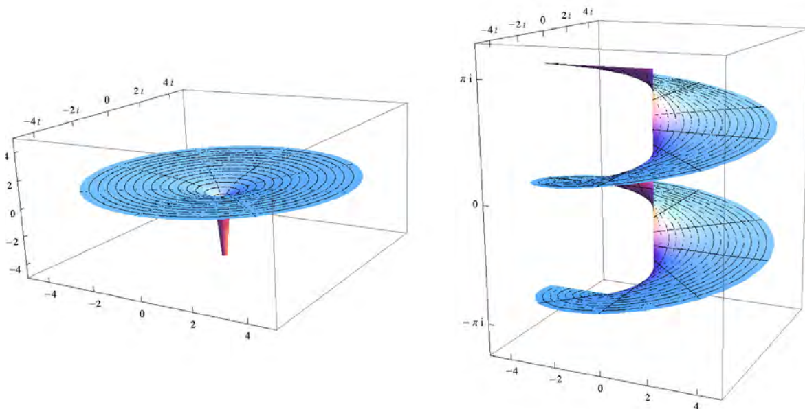
Abbildung 2.7: Der Realteil und Imaginärteil zum mehrwertigen „ z \mapsto \log z “.
