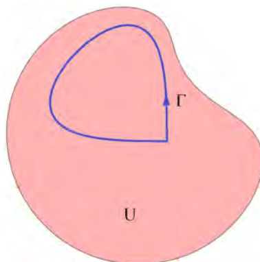
Abbildung 11.2: U , \Gamma und die Richtung von \gamma
