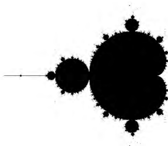
Abbildung 3.4: Ein Bild zur Mandelbrot-Menge, früher mal hergestellt durch ein Java-applet auf https://www.h-schmidt.net/MandelApplet/mandelapplet.html .
