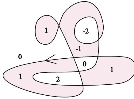
Abbildung 4.6: Die Umlaufzahlen z \mapsto n(\gamma, z) einer Kurve an verschiedenen Stellen.
