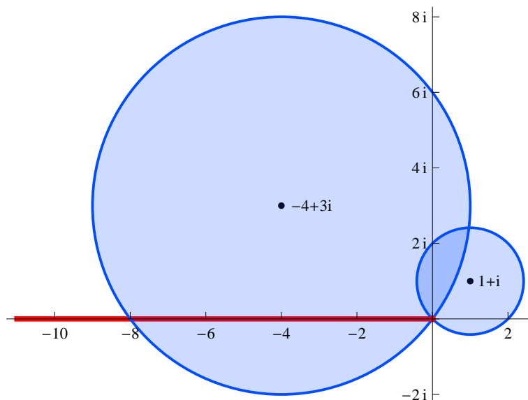
Abbildung 6.2: Definitionsgebiete von \text{Log} mit Schnitt (-\infty, 0] und von den zwei zugehörigen Potenzreihen aus Beispiel 6.4 und 6.5.
