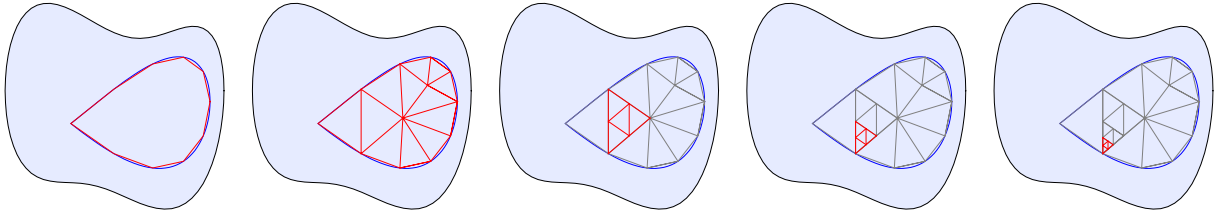
Abbildung 4.2: Einige Schritte zum Beweis des Integralsatzes: Polygonzug statt Kurve, Triangulieren, Verfeinern, Verfeinern, Verfeinern.
