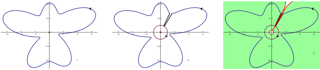
Abbildung 4.4: Links die Kurve um eine Singularität. In der Mitte derart geändert, dass die Singularität außerhalb liegt. Rechts sieht man, wie die neue Kurve innerhalb einer einfach zusammenhängenden Menge (in grün) liegt.
