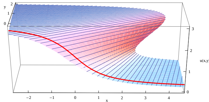
Abbildung 5.3: Skizzen der Kurven t \mapsto (x(t), y(t), U(t)) aus (5.16) bei verschiedenen s . In rot ist die Bedingung u(x, 0) = \frac{1}{2}\pi - \arctan x dargestellt.
