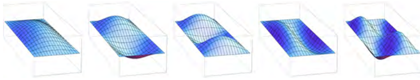
Abbildung 11.5: Darstellung der ersten 5 Eigenfunktionen aus Beispiel 11.12.
