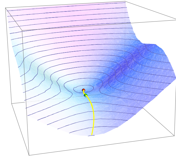
Abbildung 16.4: Lokales Minimum (rot) und ein zweiter stationärer Punkt (grün) in Dimension 2. Man sucht diesen Punkt (= Funktion für das obige Beispiel), indem man alle Wege vom roten Punkt in die Tiefe betrachtet. Auf jedem Weg \gamma gibt es ein Maximum m_\gamma . Schlussendlich nimmt man das Infimum von m_\gamma über alle Wege \gamma und versucht zu zeigen, dass dieses Infimum angenommen wird.
