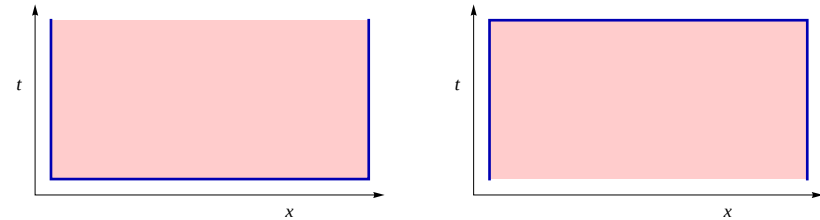
Abbildung 11.1: Schematische Darstellung vorgeschriebener Randwerte bei der Wärmeleitungsgleichung. Obwohl die Eindeutigkeit für beide Fälle gilt, heißt das noch nicht, dass beide Randwertprobleme wohldefiniert sind im Sinne von Hadamard. Mit Anfangswert u(x, 0) = u_0(x) und u_0 \in C(\bar{\Omega}) kann man Existenz und Robustheit zeigen. Für u(x, T) = u_1(x) und u_1 \in C(\bar{\Omega}) gilt dies nicht.
