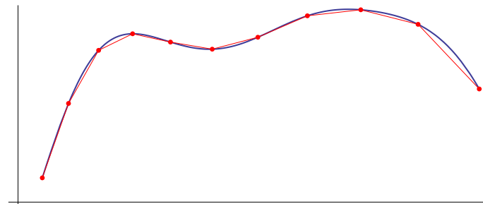
Abbildung 2.6: Bogenlänge wird approximiert mittels Polygonzug
