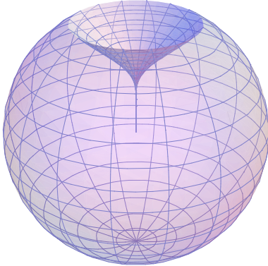
Abbildung 14.2: Bild einer Kugel mit einem „Lebesgue thorn“. Das Horn (oder der Dorn) ist hier wie folgt definiert: D = \{(x, y, z) : x^2 + y^2 < \exp(-1/z) \text{ für } z > 0\} . Also gilt \Omega = B_1(0) \setminus D .
