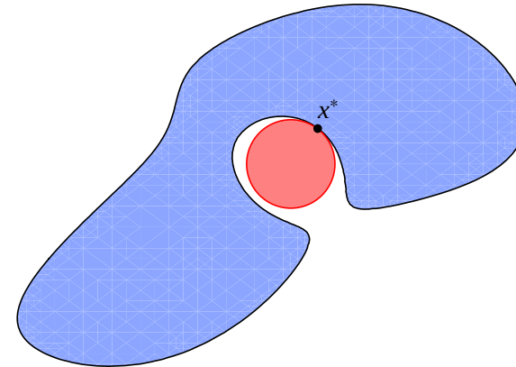
Abbildung 14.1: Die äußere Kugelbedingung.
