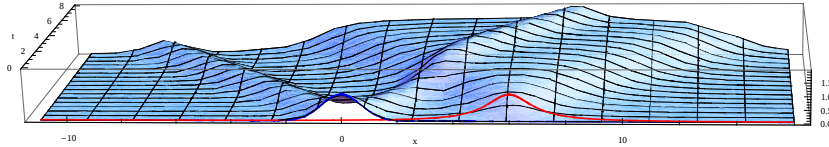
Abbildung 7.1: Skizze der Lösung nach d'Alembert von (7.2) mit c = 1 und u_0(x) = e^{-x^2} (in blau) und v_0(x) = \frac{1}{1+(x-6)^2} (in rot).
