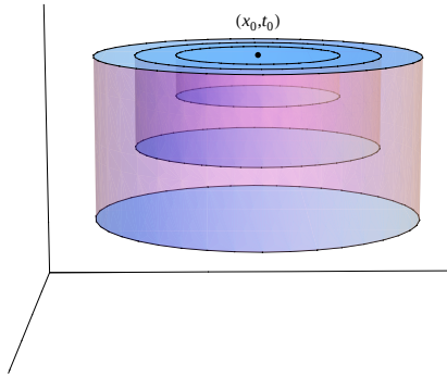
Abbildung 11.2: Die Zylinder Z_1 \supset Z_2 \supset Z_3 aus dem Beweis zu Theorem 11.6.
